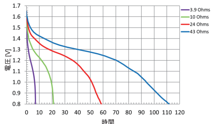
定抵抗放電
