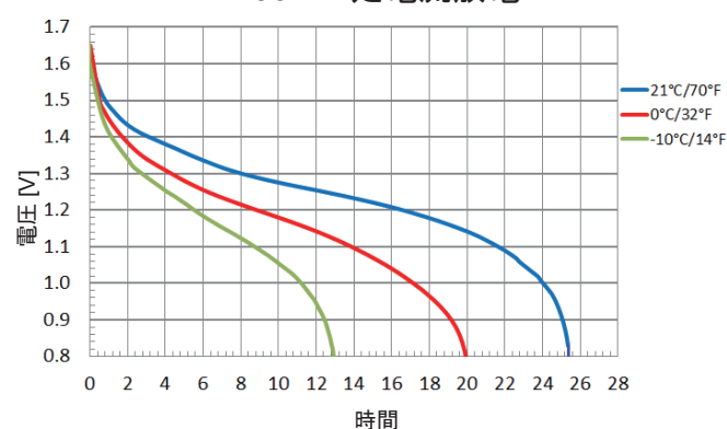
100mA 定電流放電
