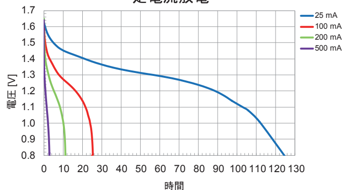
定電流放電
