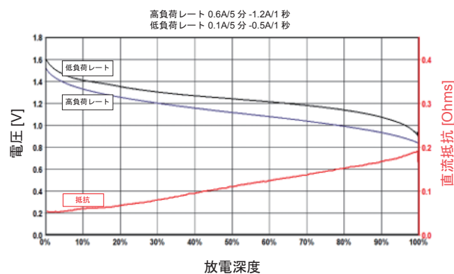
公称内部抵抗
