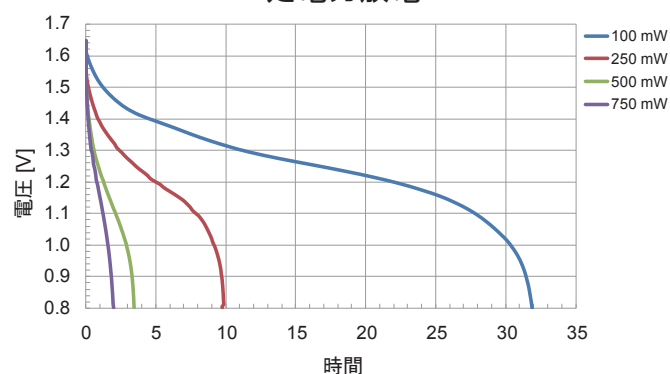
定電力放電
